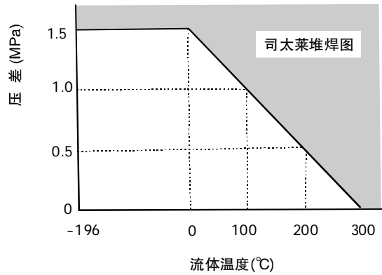
图4 司太莱堆焊的工作范围
