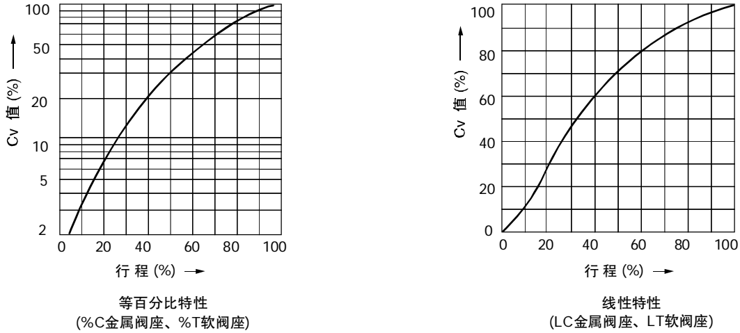
图1 大容量流量特性曲线
