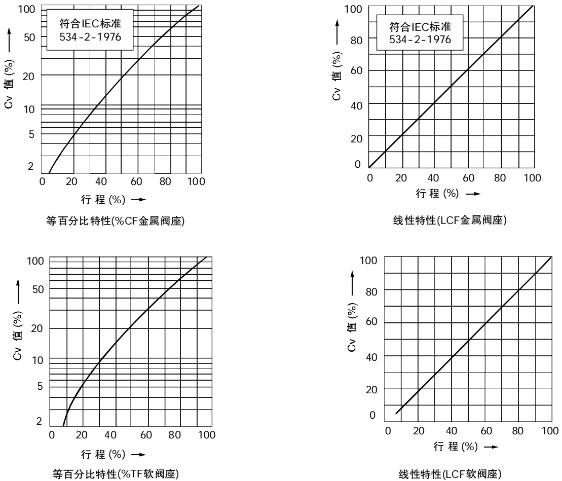
图2 高精度流量特性曲线
